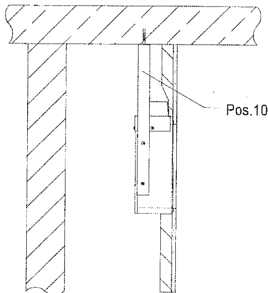
Deckenmontage
